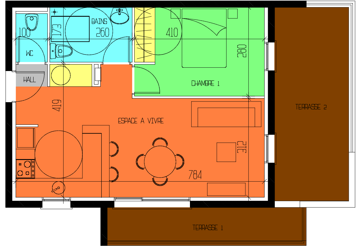
PLAN DU LOGEMENT
